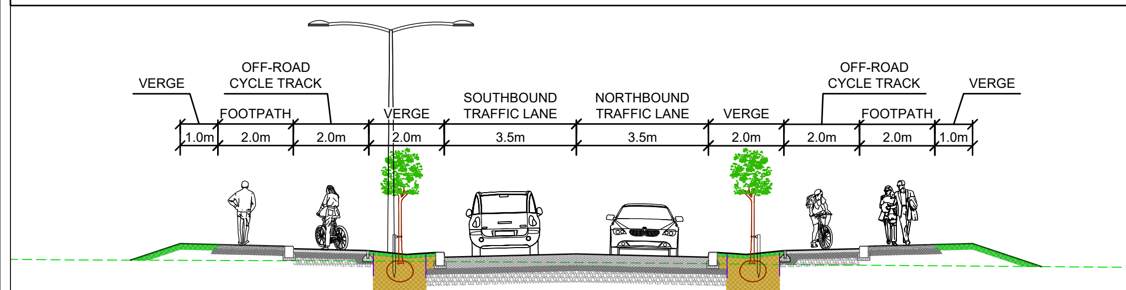
Section D-D (Scale: 1:100)
