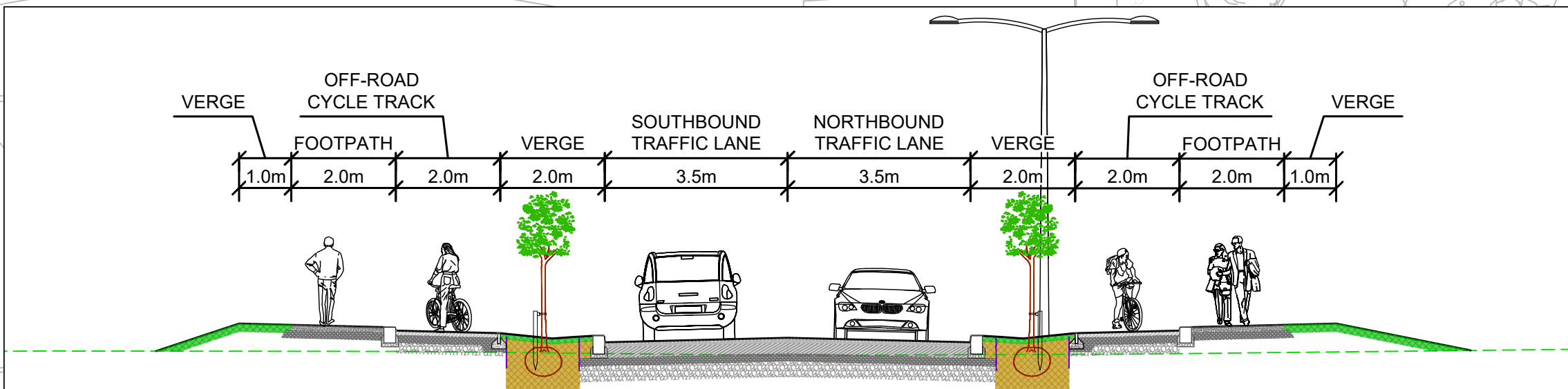
Section C-C (Scale: 1:100)
